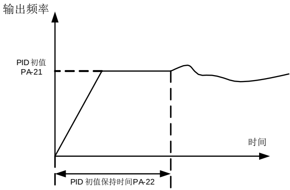
图 6-27 为 PID 初值的功能示意 图。
