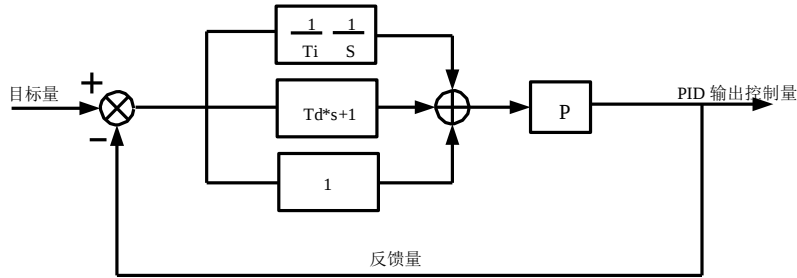
图 6-25 过程 PID 原理框图
