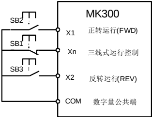
图 6-8 三线式控制模式 1
