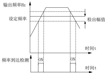
图 6-17 频率到达检出幅值示意图
