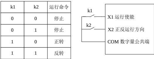
图 6-7 两线式模式 2
