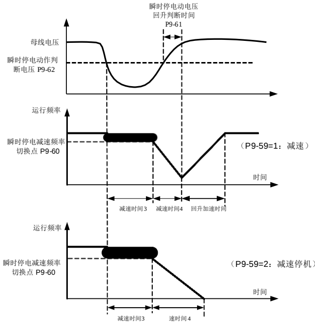
图 6-24 瞬时停电动作示意图
