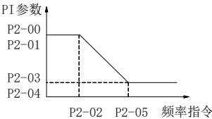
图 6-2 PI 参数示意图
