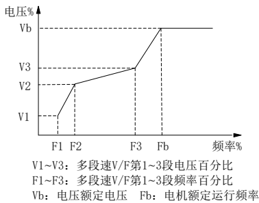
图 6-4 多点 V/F 曲线设定示意图
