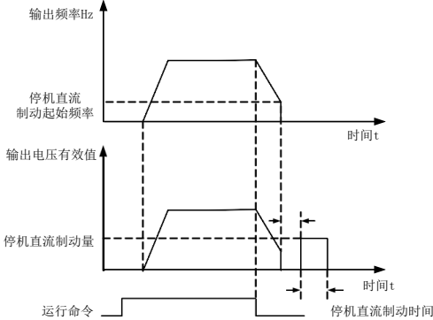
图 6-13 停机直流制动示意图
