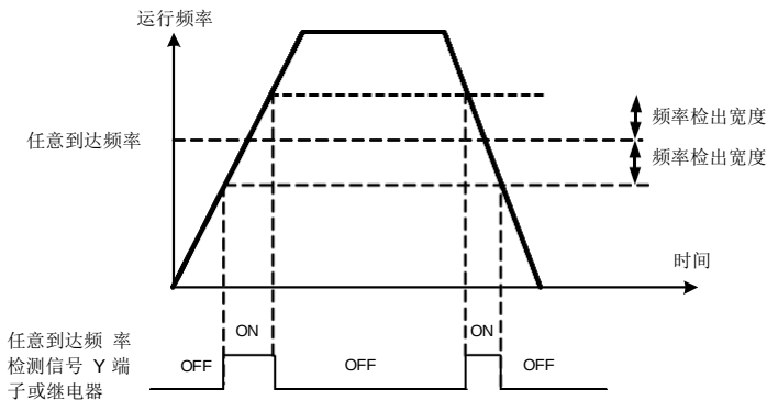
图 6-20 任意到达频率检测示意图
