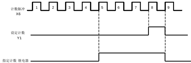
图 6-29 设定计数值给定和指定计数值给定示意图
