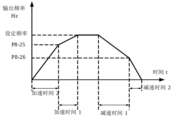
图 6-19 加减速时间切换示意图
