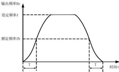
图 6-12 S 曲线加减速 B 示意图
