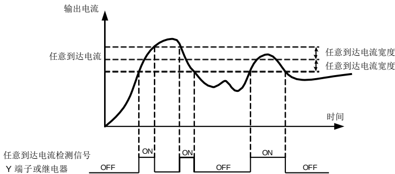
图 6-23 任意到达电流检测示意图
