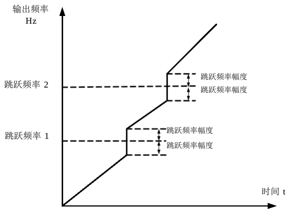
图 6-18 加减速过程中跳跃频率有效示意图
