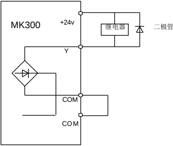
图 3-17 数字输出端子接线示意图
