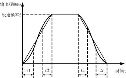
图 6-11 S 曲线加减速 A 示意图
