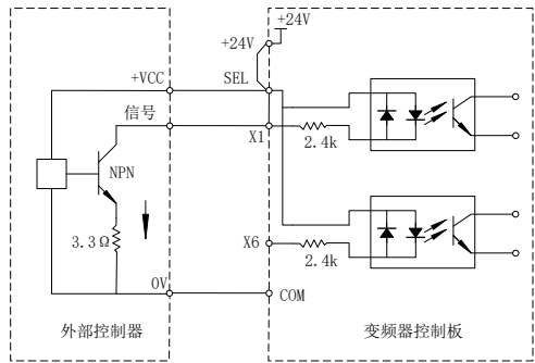
图 3-15 漏型接线方式
