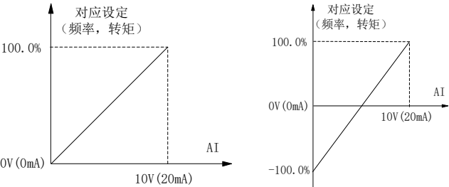
图 6-10 模拟给定与设定量的对应关系
