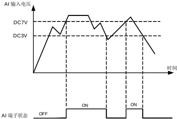
图 6-31 AI 端子有效状态判断
