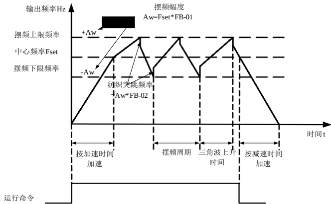
图 6-28 摆频工作示意图
