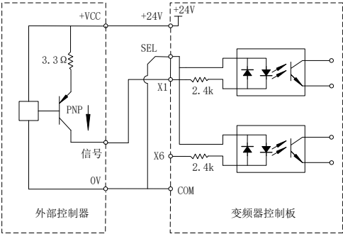
图 3-16 源型接线方式
