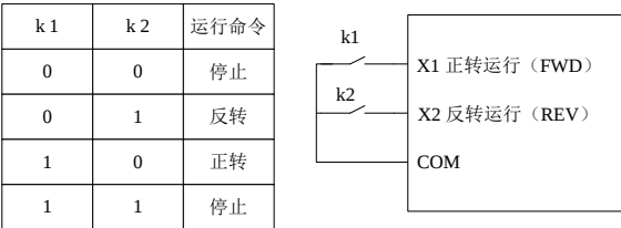
图 6-6 两线式模式 1
