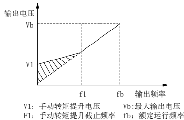
图 6-3 手动转矩提升示意图
