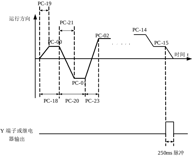
图 6-30 简易 PLC 示意图
