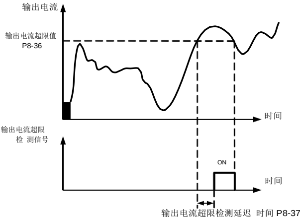
图 6-22 输出电流超限检测示意图
