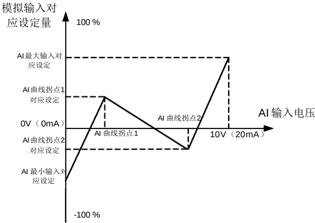
图 6-32 曲线 4 和曲线 5 示意图
